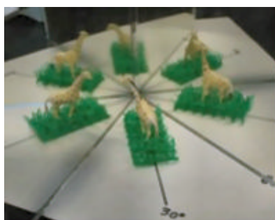
2枚の鏡を60°に
