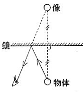
鏡に映る像
