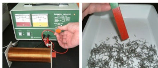
鋼製磁石を入れたコイルに交流をかけ、電圧を下げていくと磁力を消せる。
