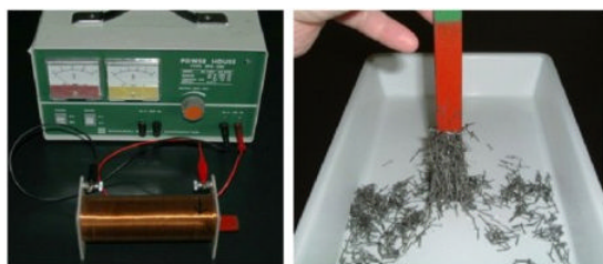
鋼製磁石を入れたコイルに直流を流すと磁力が増す。
